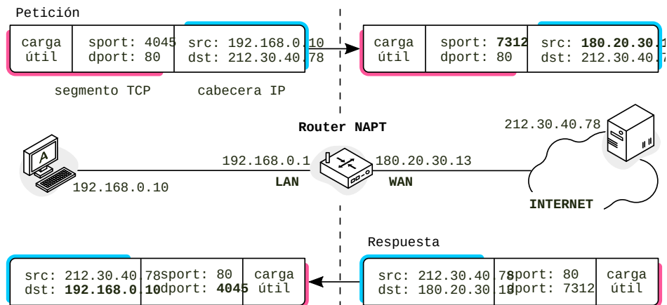
FIGURA 20.7: Ejemplo de NAPT con puertos mapeados
